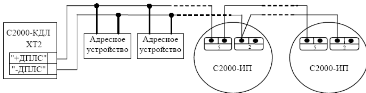
Рисунок 1 Схема соединений
