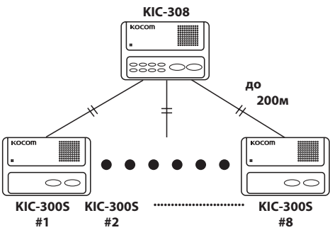
Схема подключения KIC-300S и KIC-308
