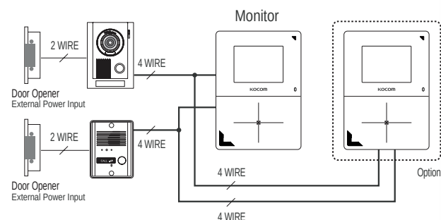
Схема подключения KCV-401EV
