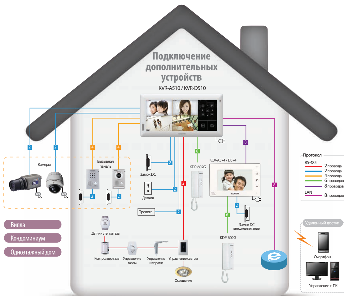
Схема подключения дополнительных устройств KVR-A510
