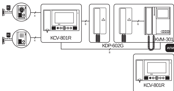
Схема подключения KCV-801R
