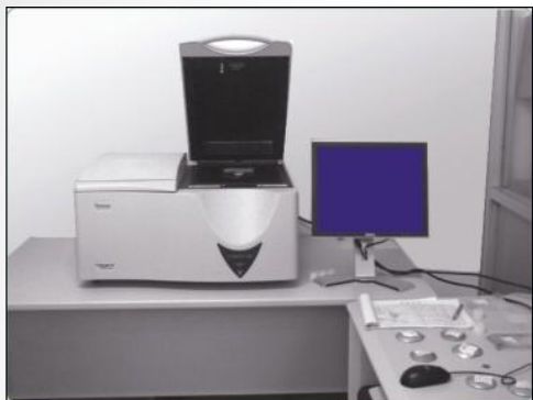
Прибор для тестирования на соответствие RoHS
